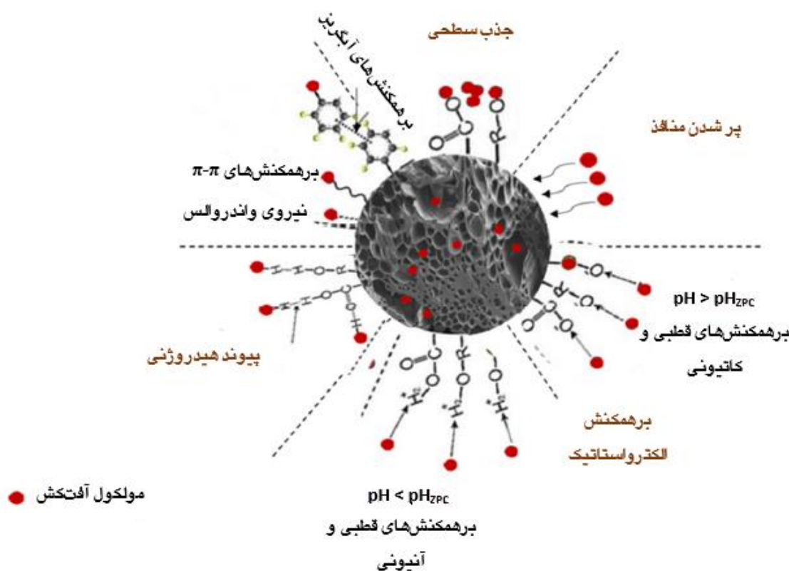
شکل ۳- سازوکارهای جذب آفتکش‌ها روی بیوچار (Cara et al., 2022).
